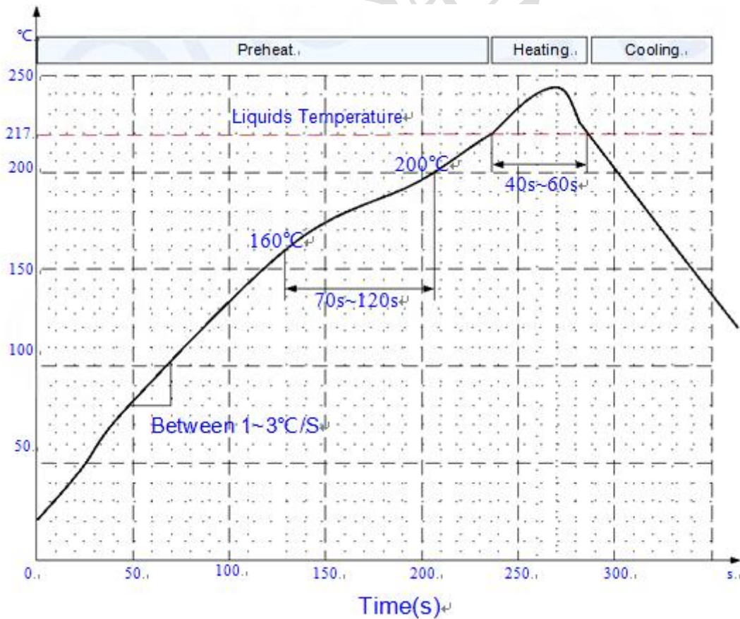
图表 21: 炉温曲
